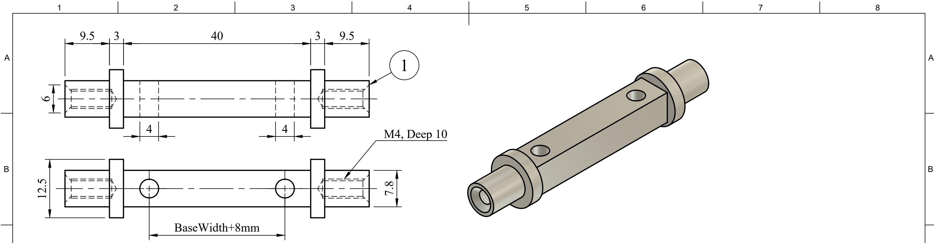
Spinder 2:1
