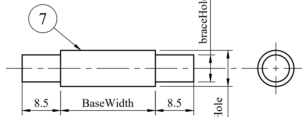
Pin 2:1
