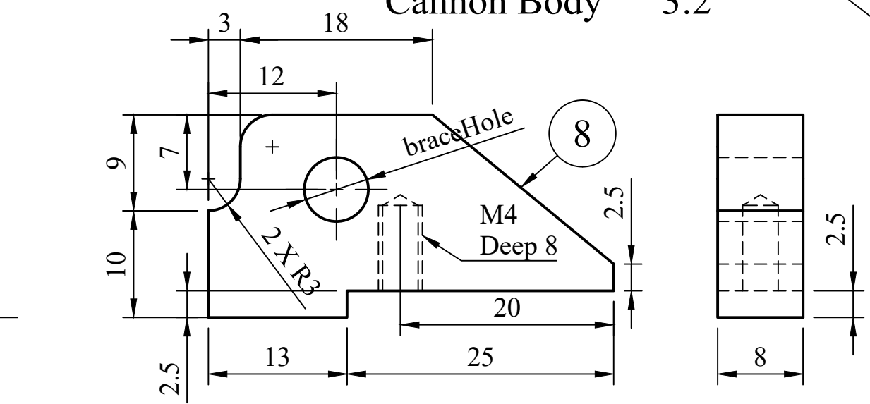
Brace 2:1
